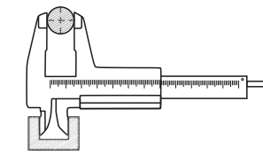
Наружный \varnothing / Outside \varnothing / Średnica zewnętrzna
